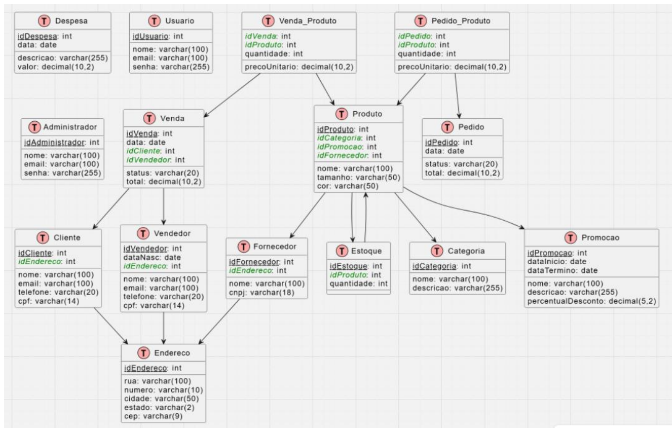
Figura 8 - Diagrama de Classes do Sistema – Modelo Lógico
